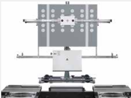
SCT 1415 v kombinaci s modulem čárového laseru (obr. kalibr. tabule pro Mercedes-Benz)
